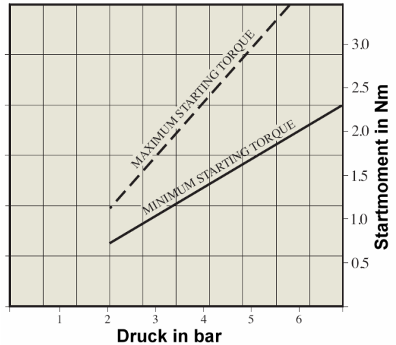
Startmoment / Druck
