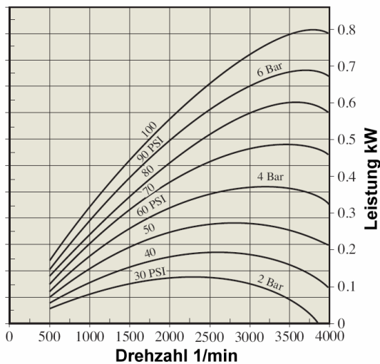
Leistung / Drehzahl
