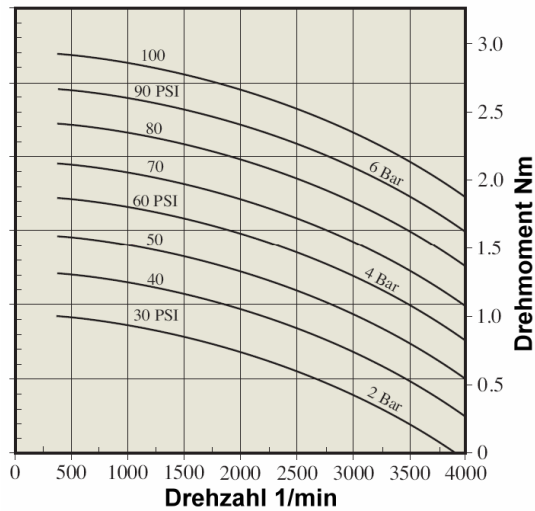
Drehmoment / Drehzahl
