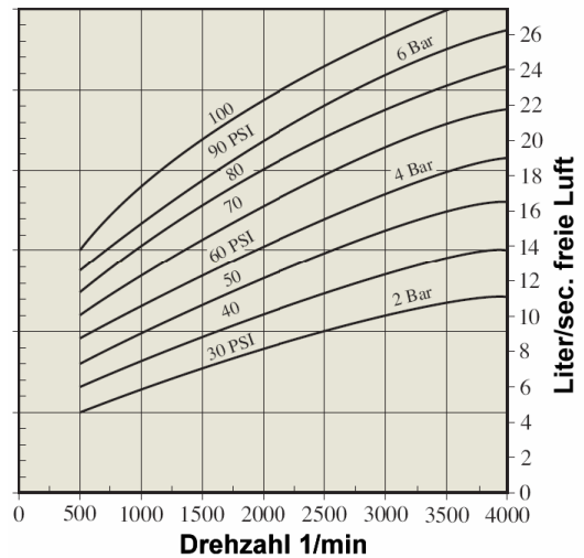
Luftverbrauch / Drehzahl
