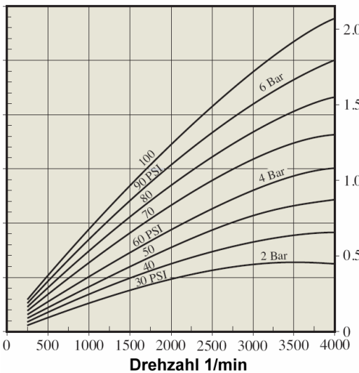
Leistung / Drehzahl
