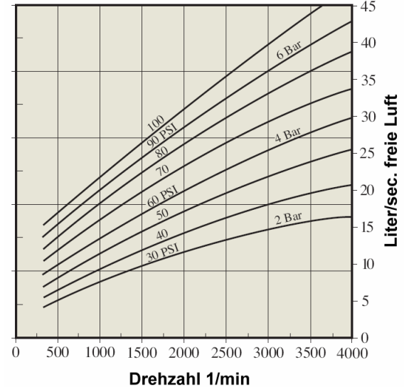
Luftverbrauch / Drehzahl
