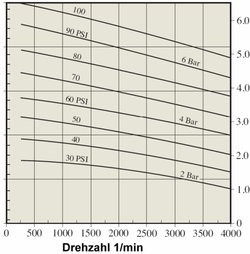
Drehmoment / Drehzahl
