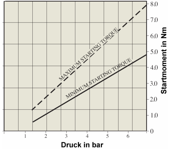
Startmoment / Druck
