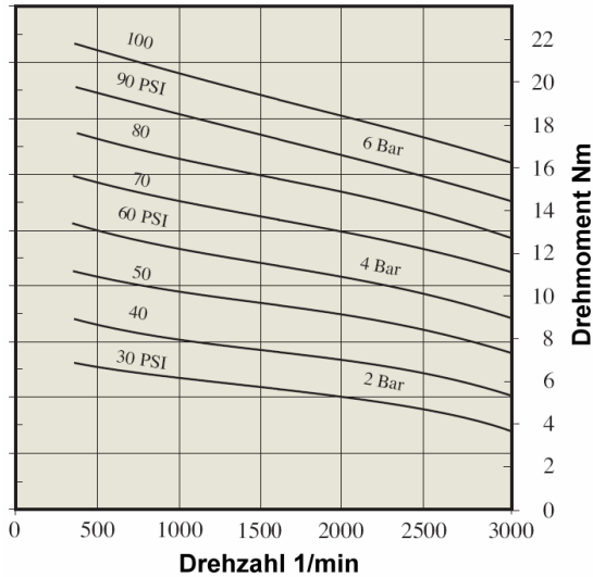
Drehmoment / Drehzahl
