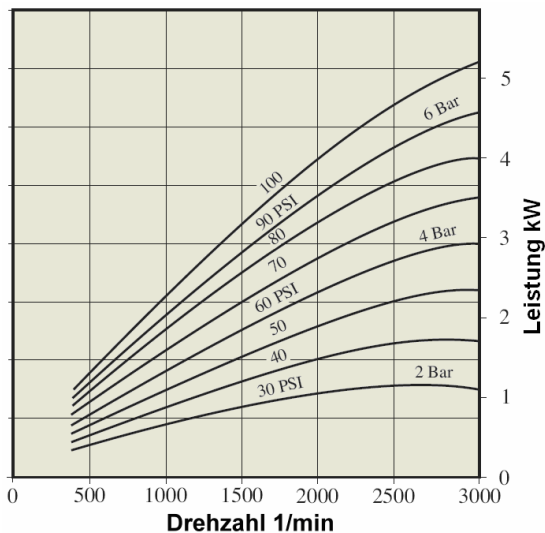
Leistung / Drehzahl
