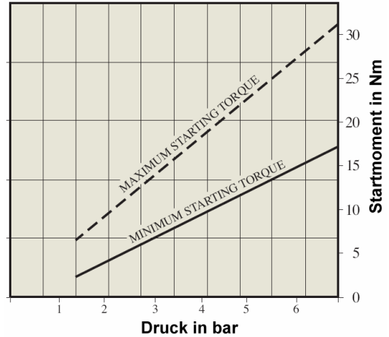
Startmoment / Druck
