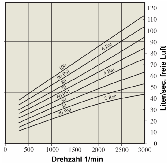
Luftverbrauch / Drehzahl
